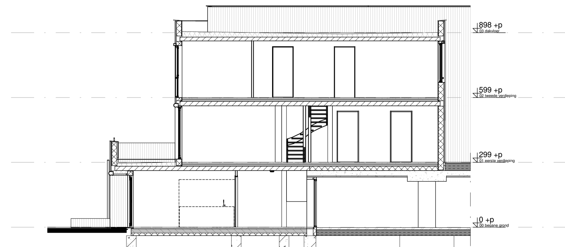
Doorsnede
