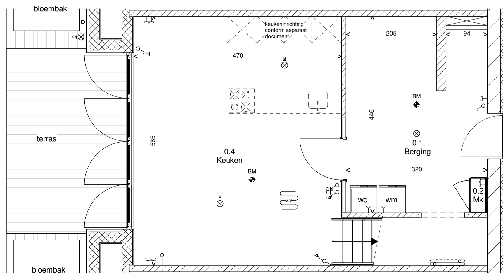
Begane grond
