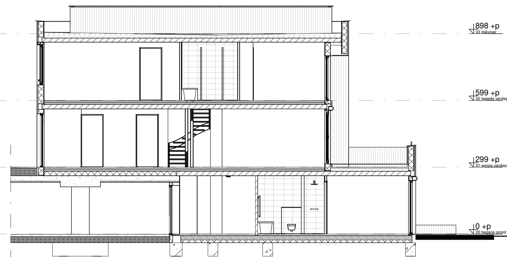
Doorsnede
