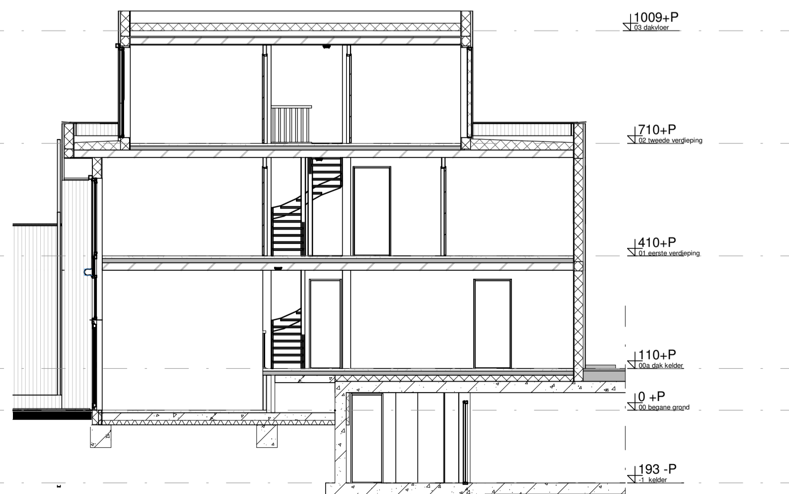
Doorsnede
