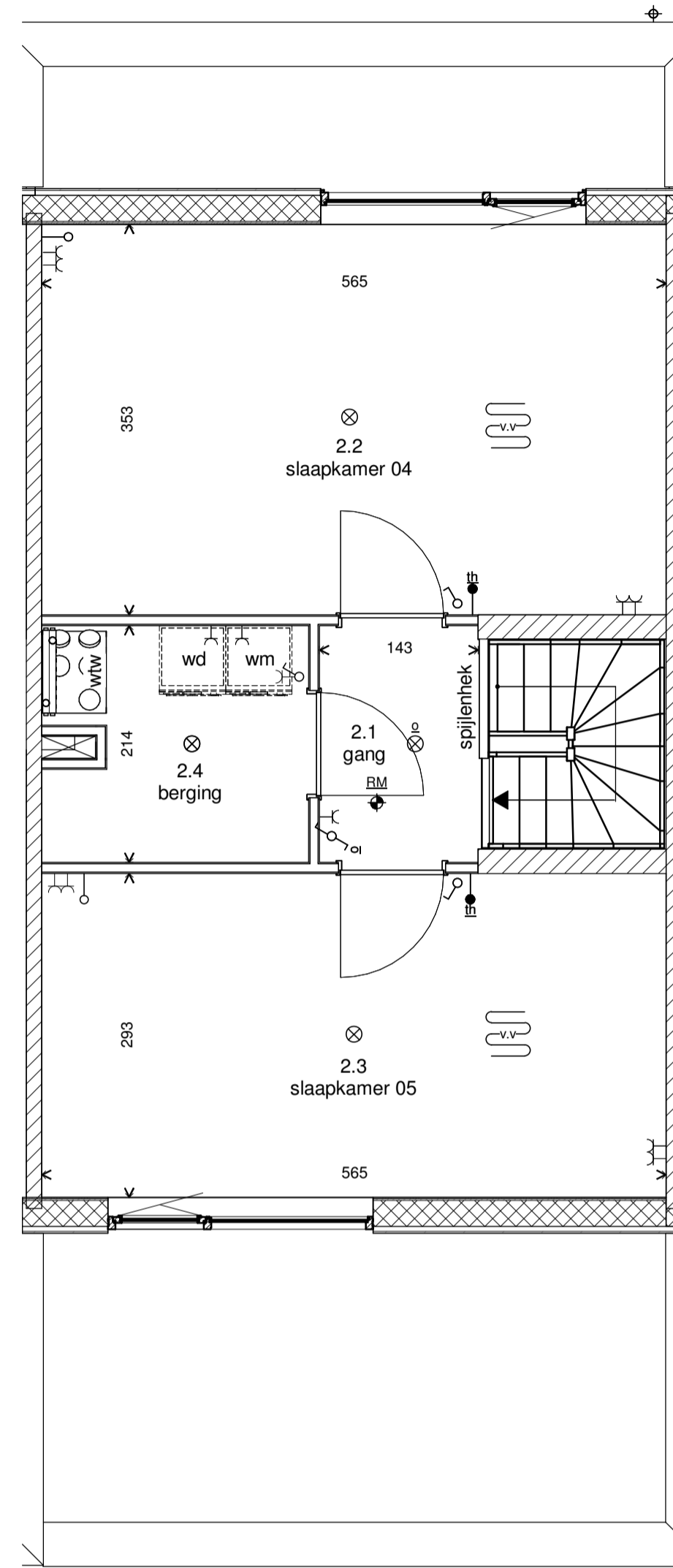
Tweede verdieping
