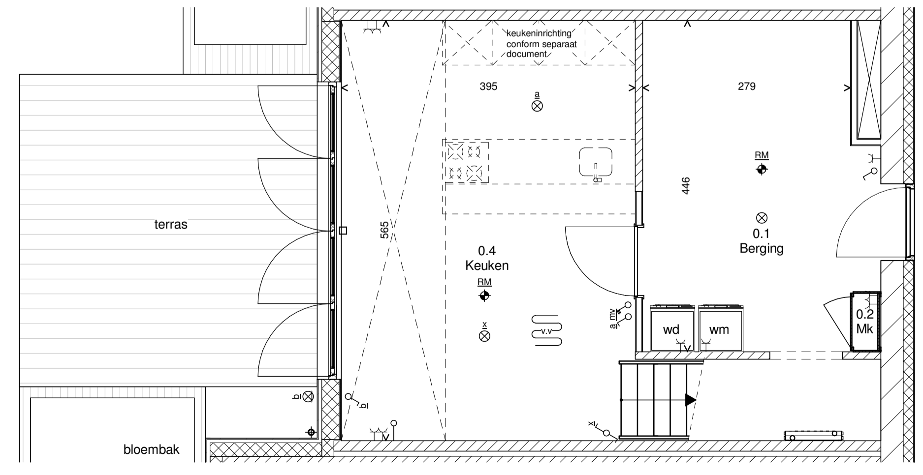
Begane grond schaal 1:50
