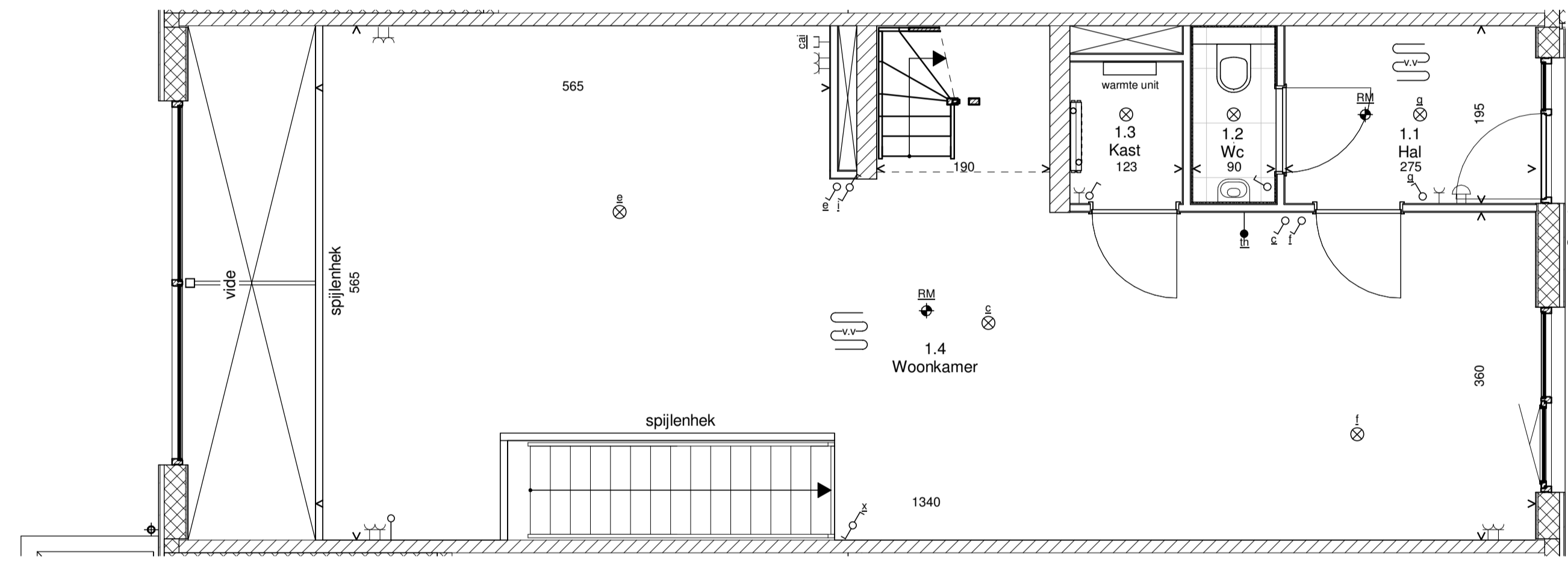
Eerste verdieping schaal 1:50
