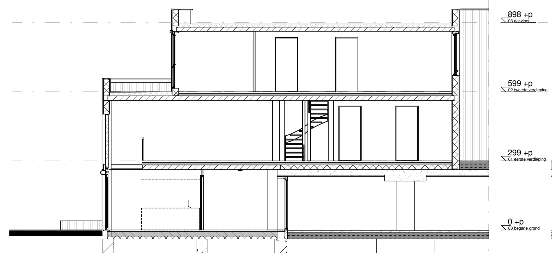
Doorsnede schaal 1:100
