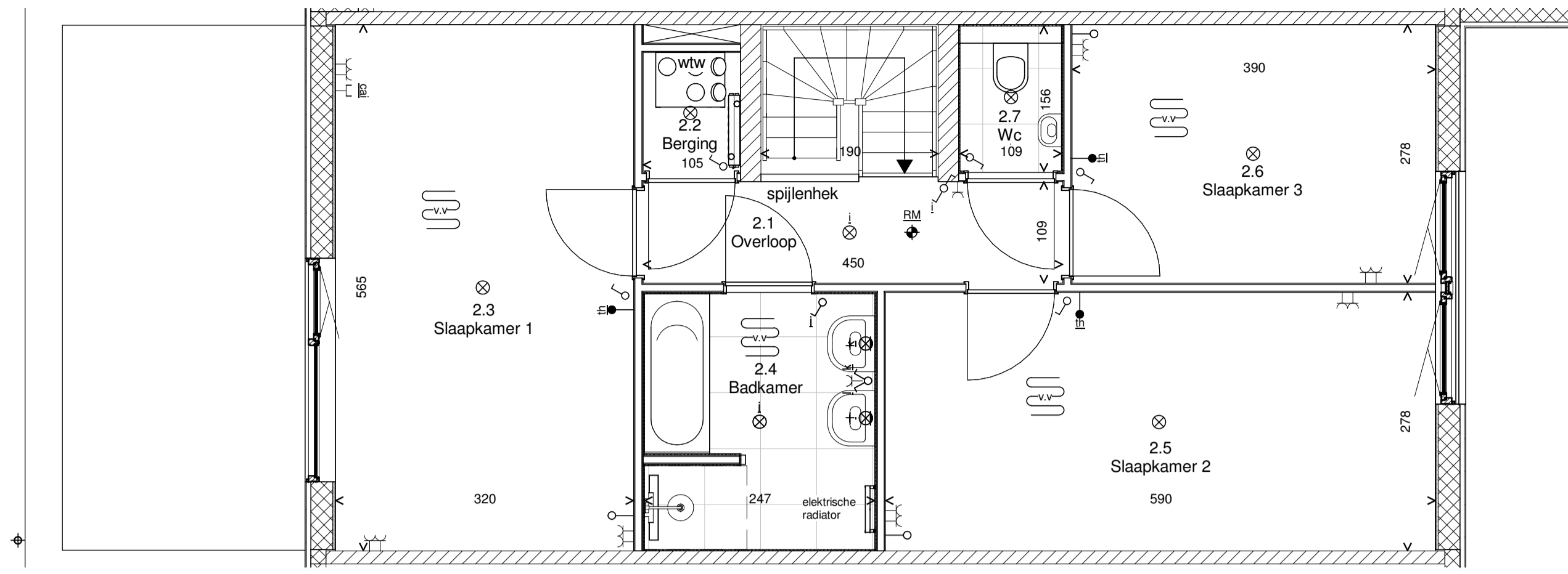
Tweede verdieping schaal 1:50
