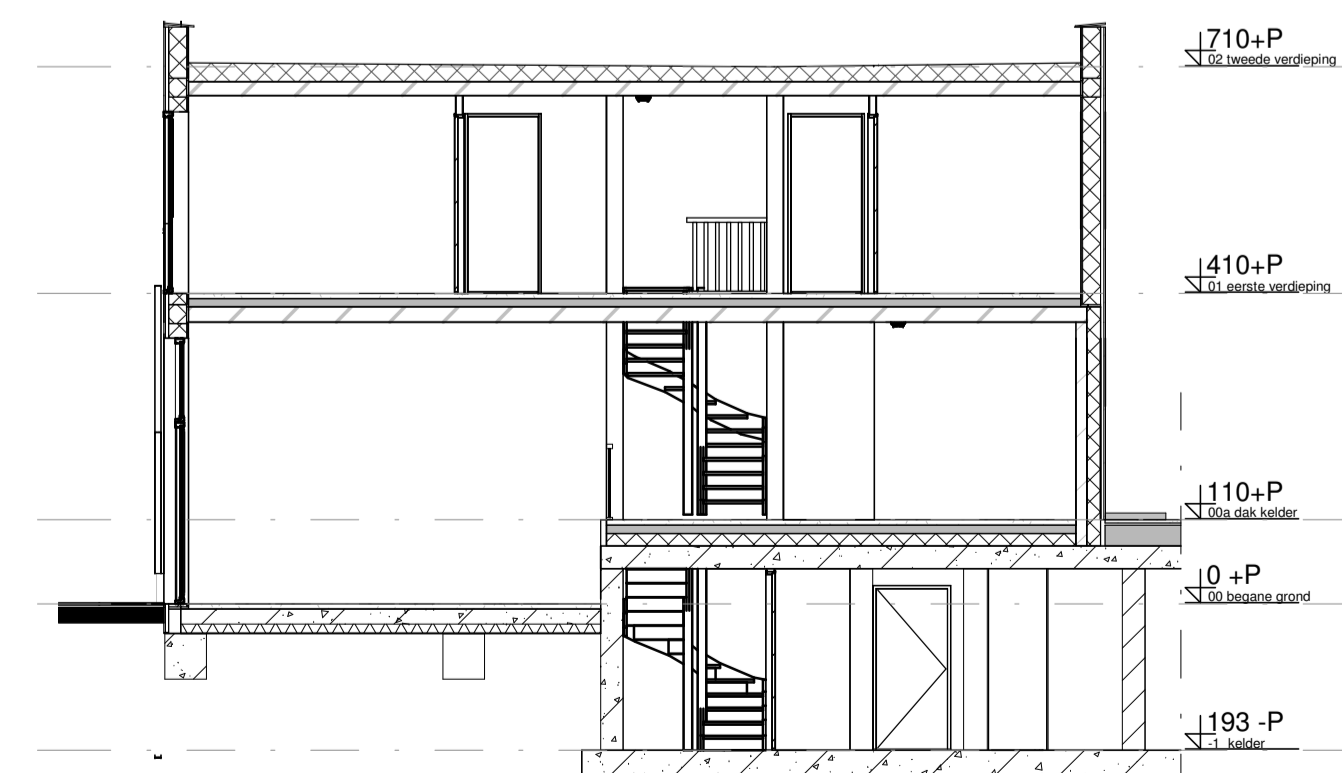
Doorsnede
