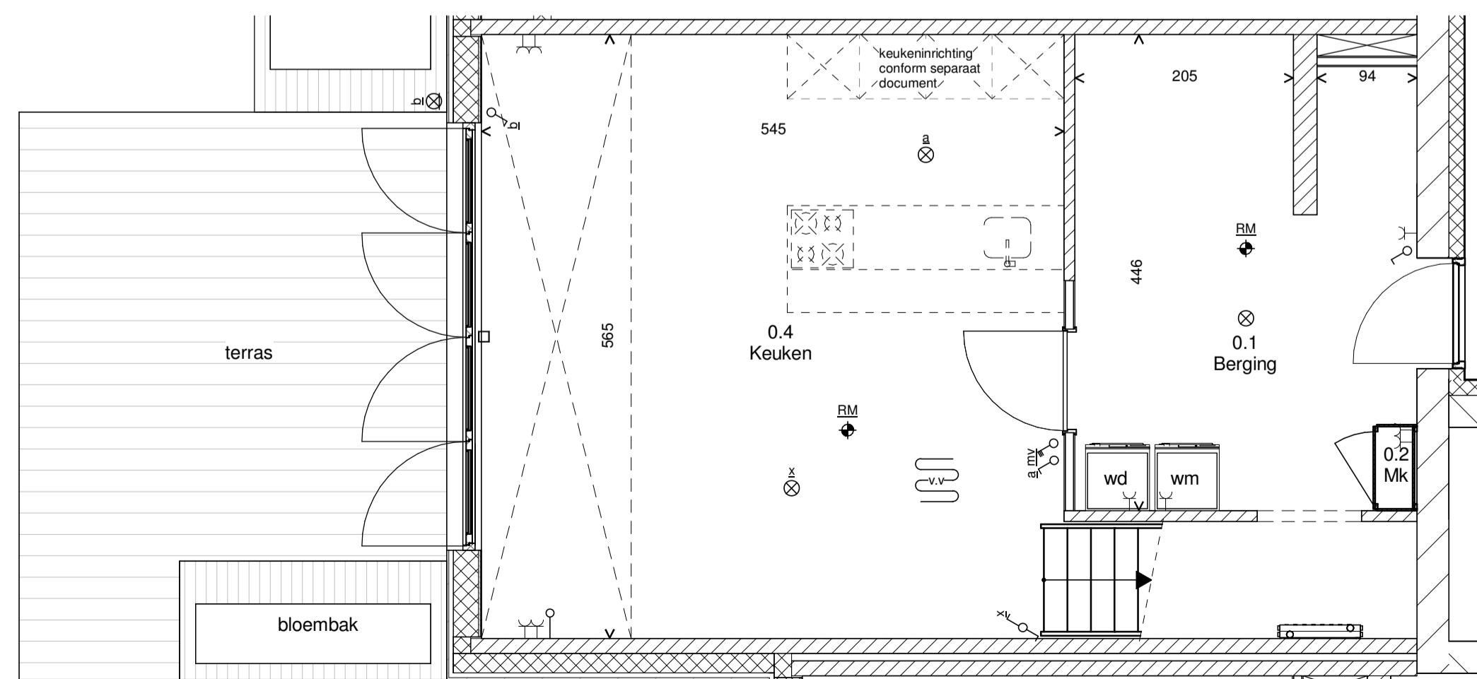
Begane grond
