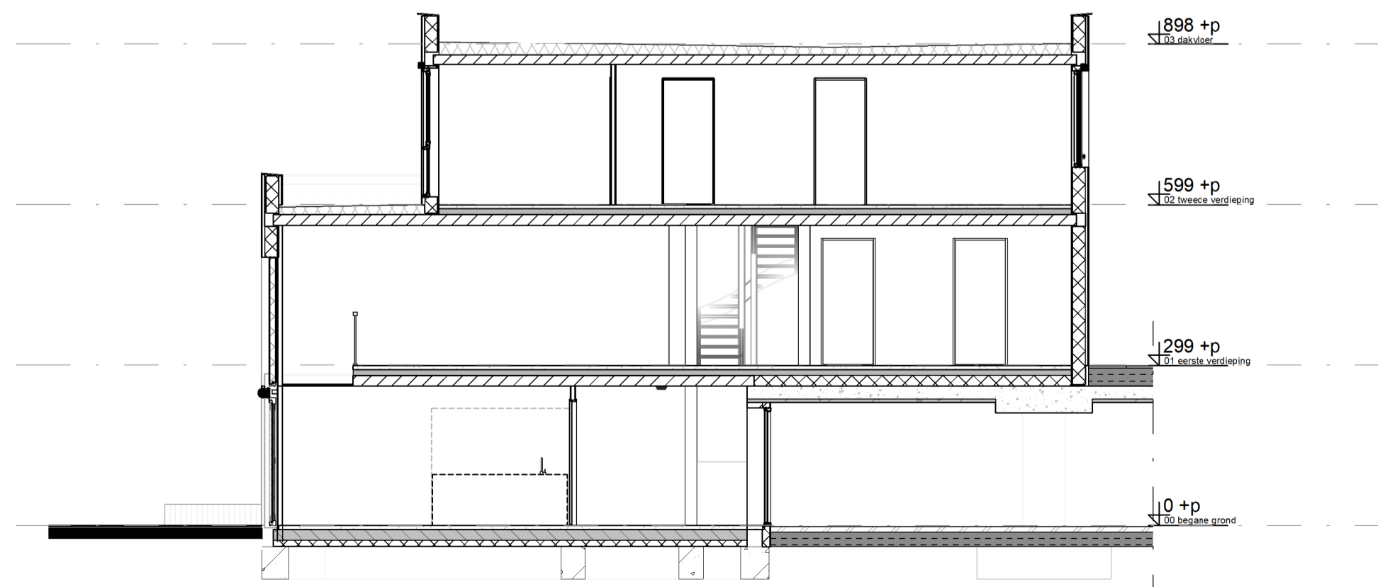
Doorsnede
