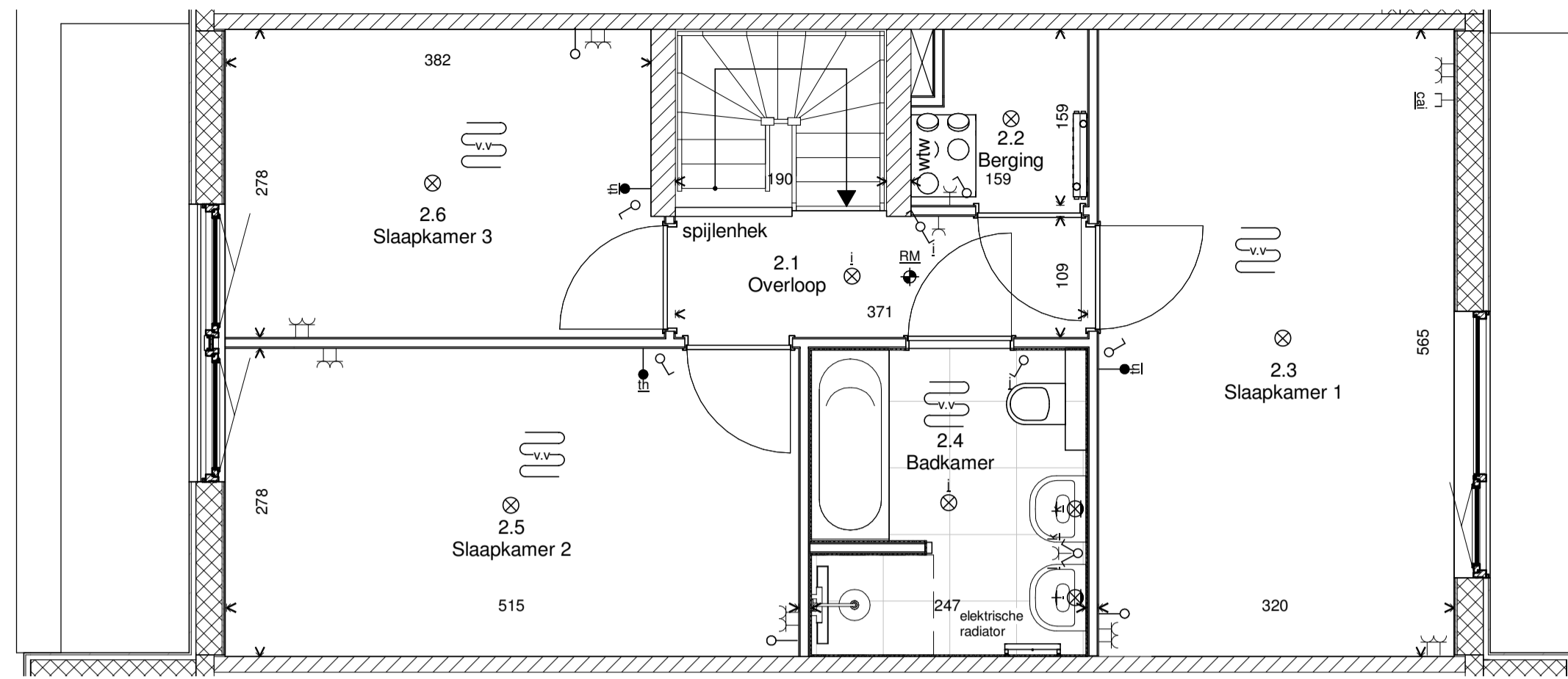
Tweede verdieping
