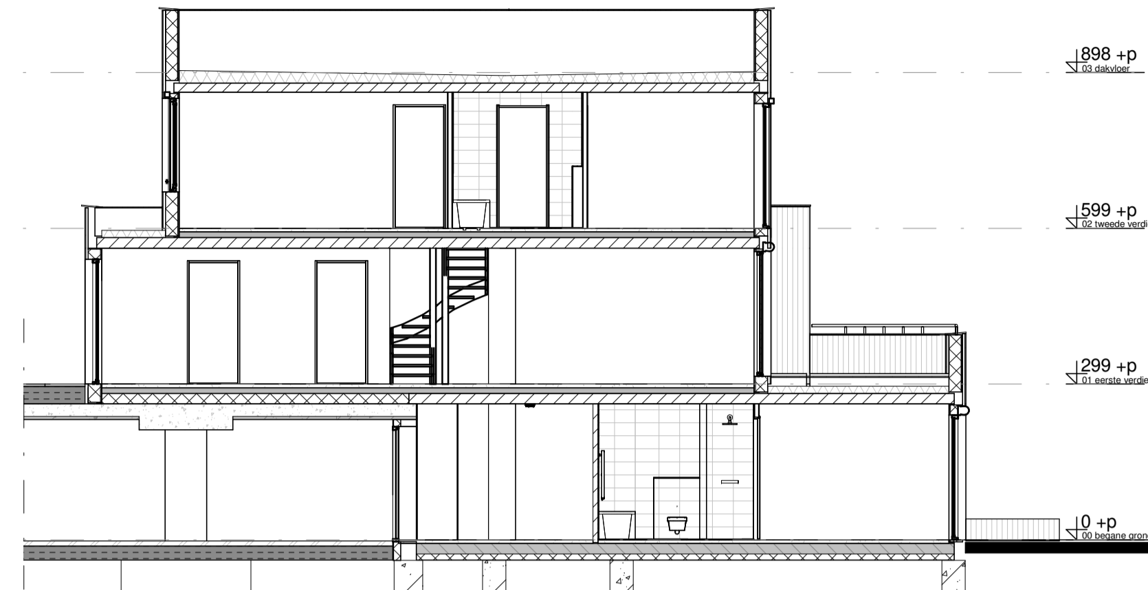
Doorsnede
