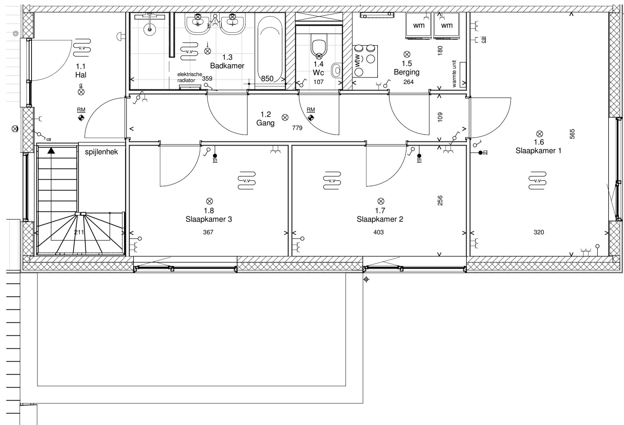
Eerste verdieping
