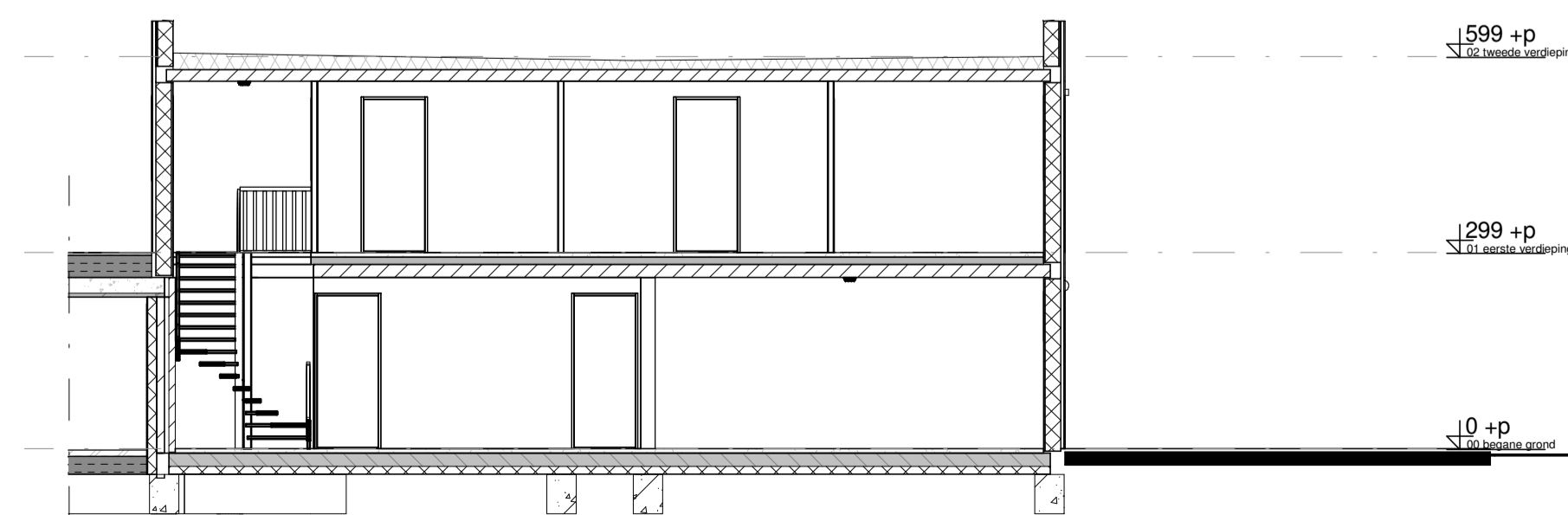
Doorsnede
