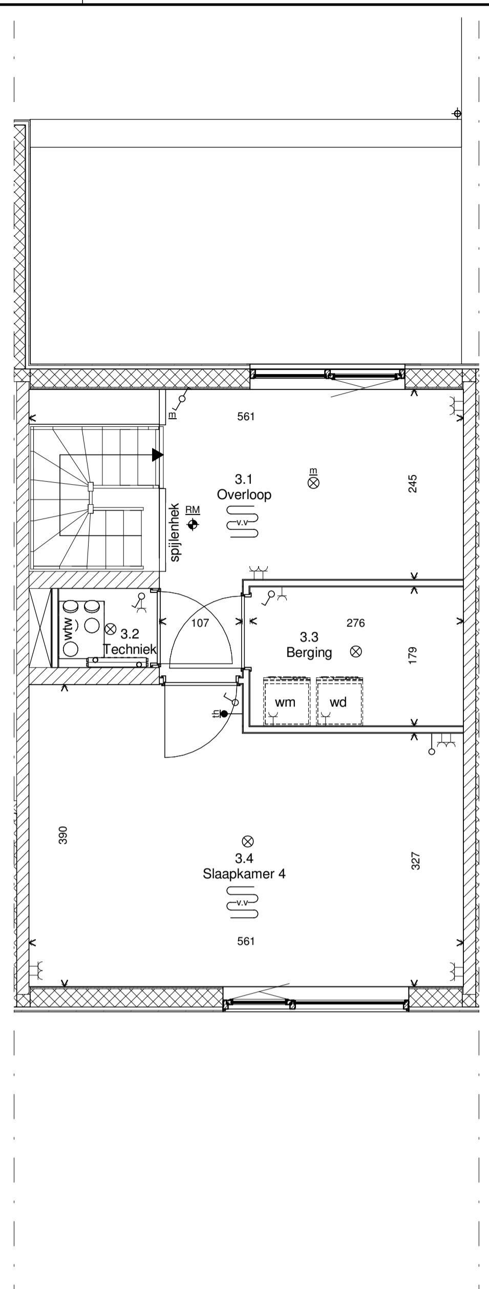
Derde verdieping schaal 1:50
