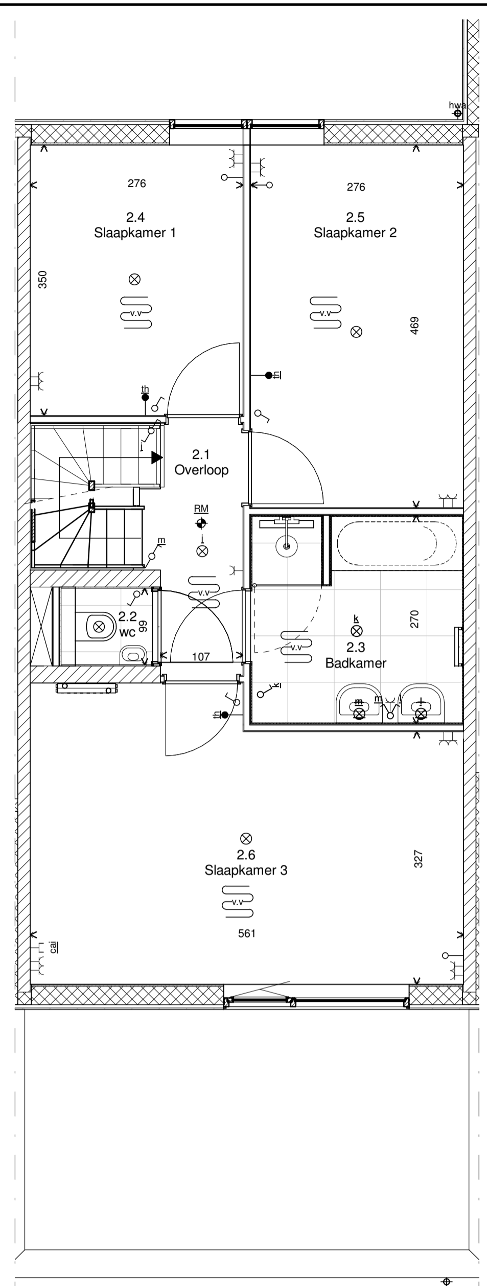
Tweede verdieping schaal 1:50
