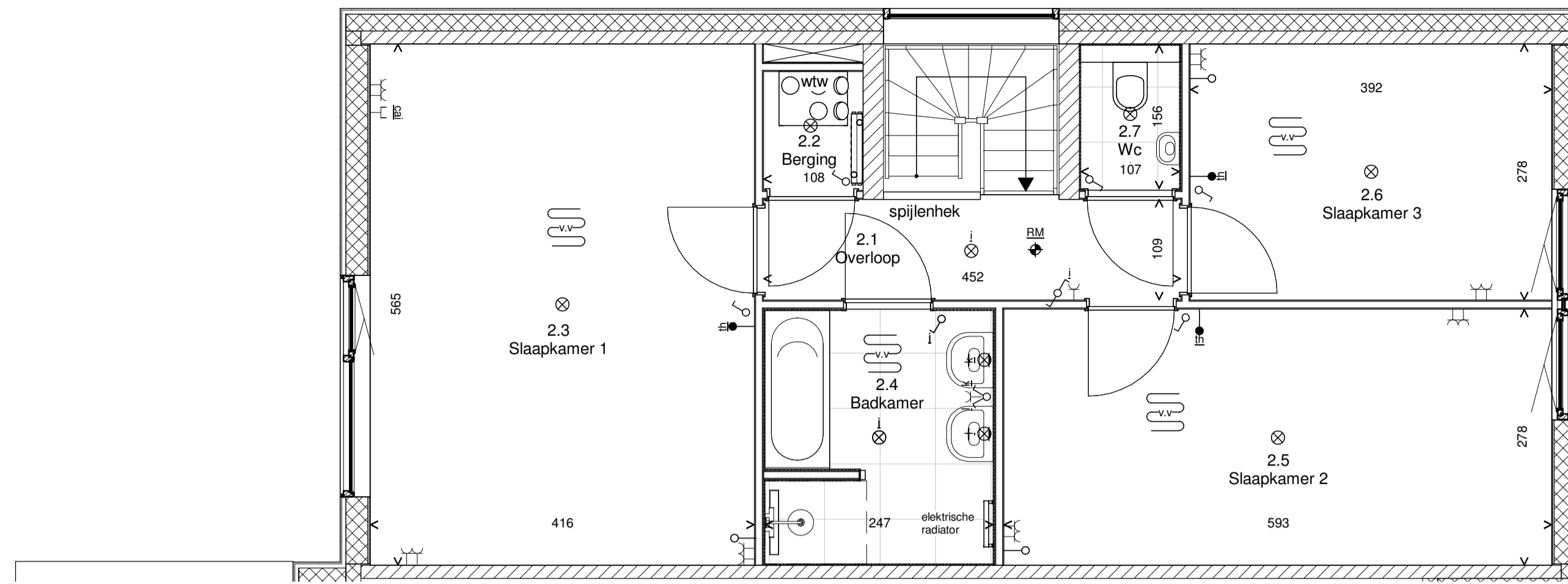
Tweede verdieping
