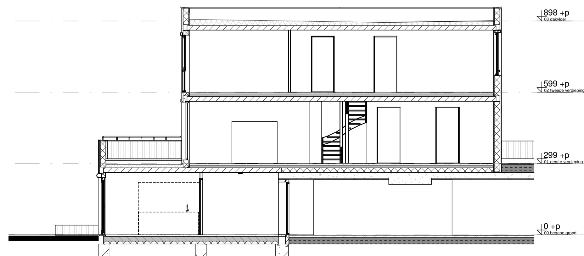
Doorsnede
