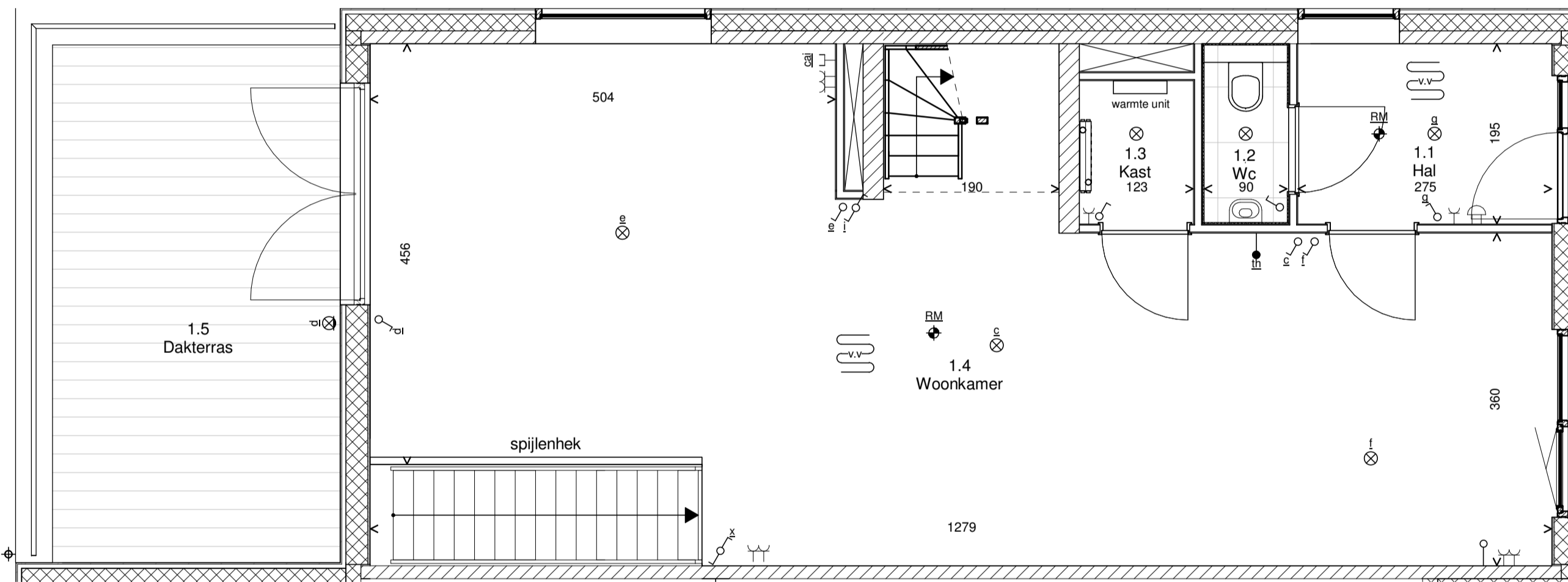
Eerste verdieping
