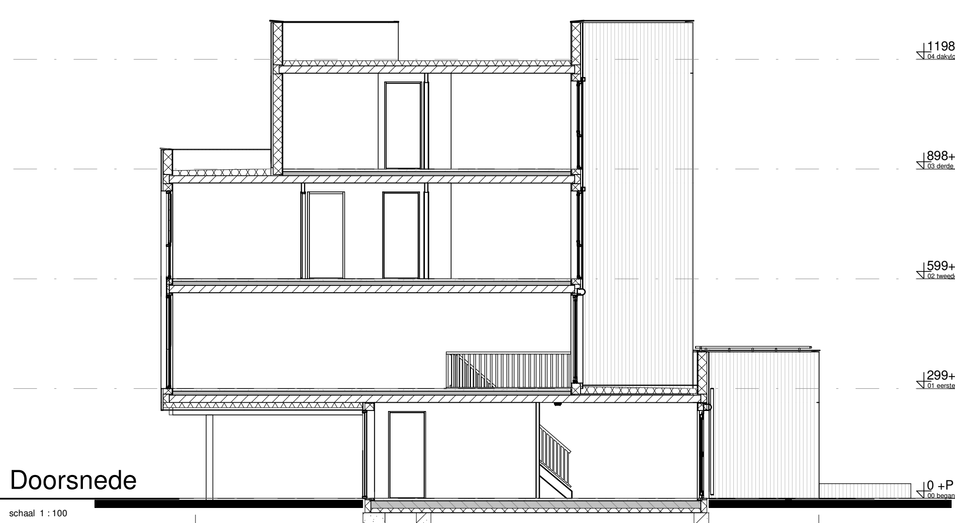
Doorsnede schaal 1 : 100
