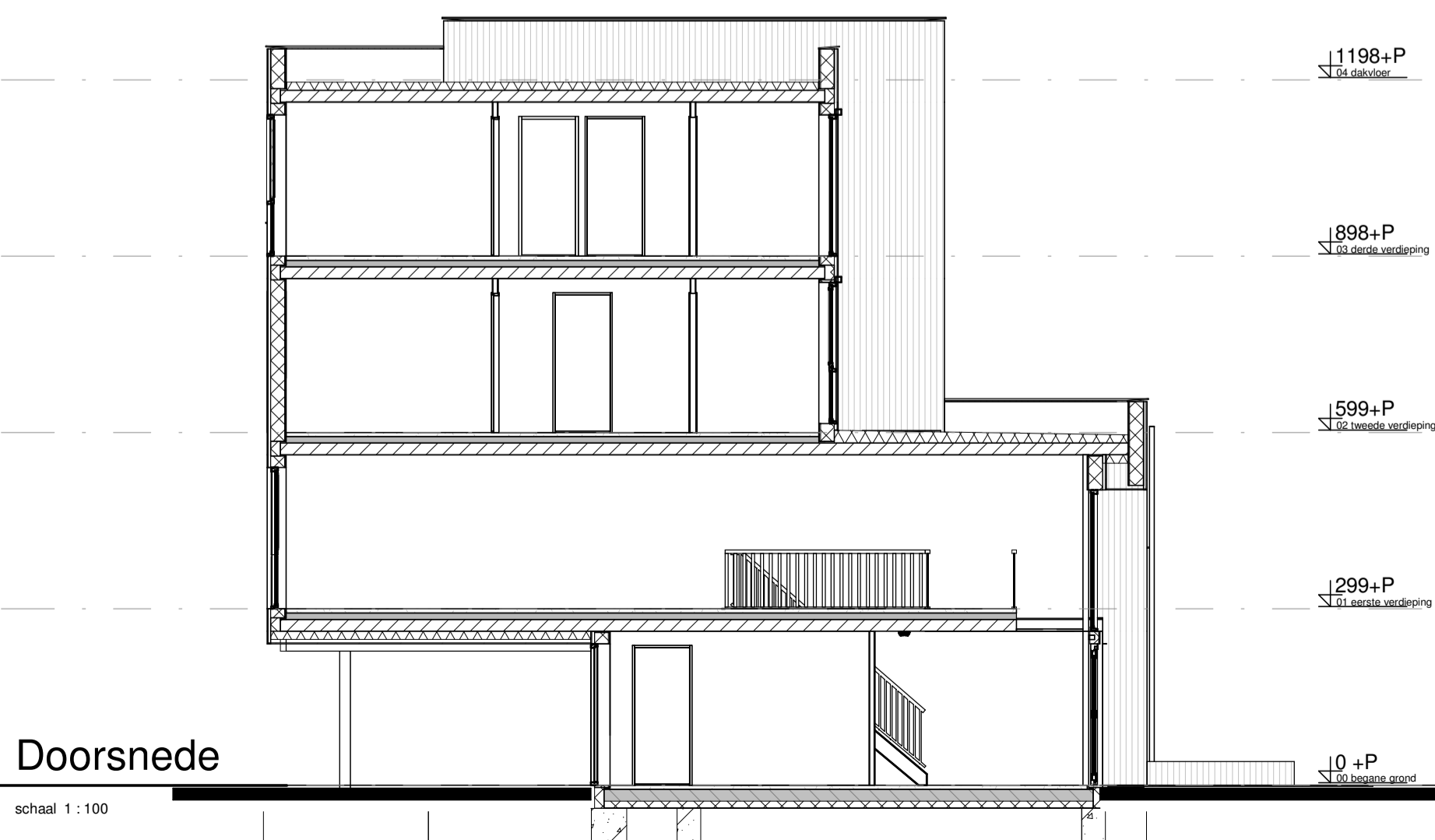
Doorsnede schaal 1 : 100
