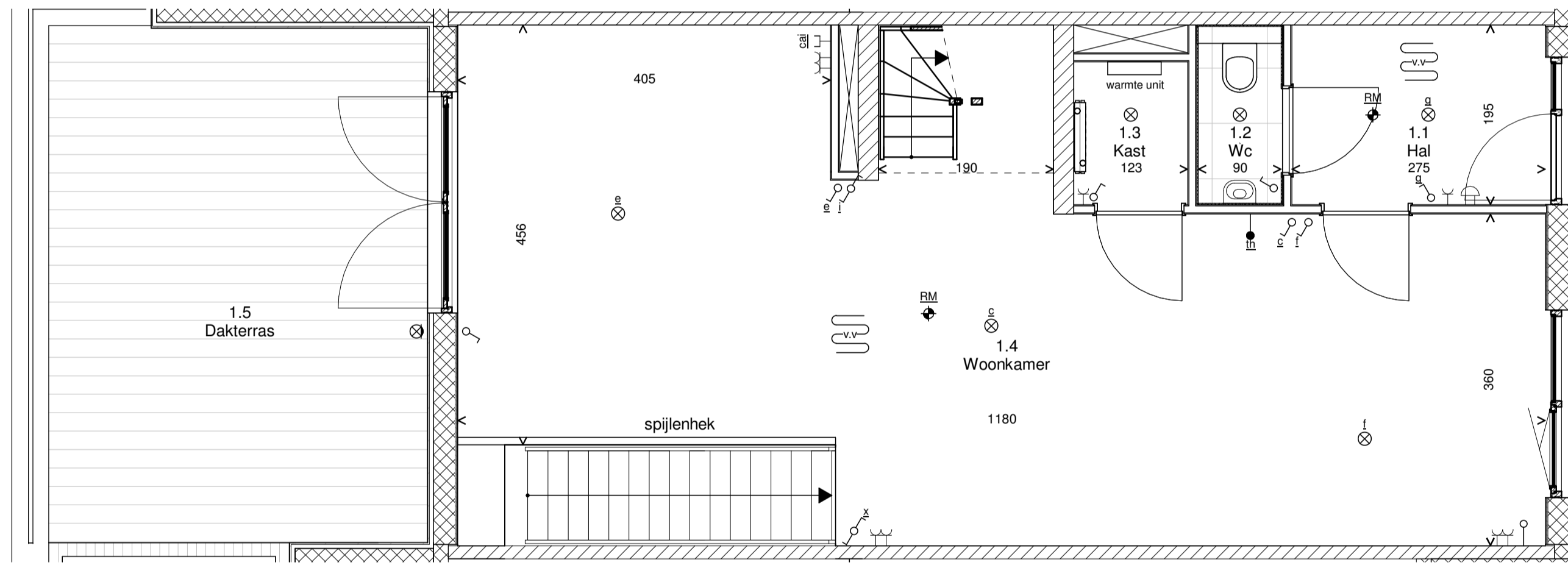
Eerste verdieping
