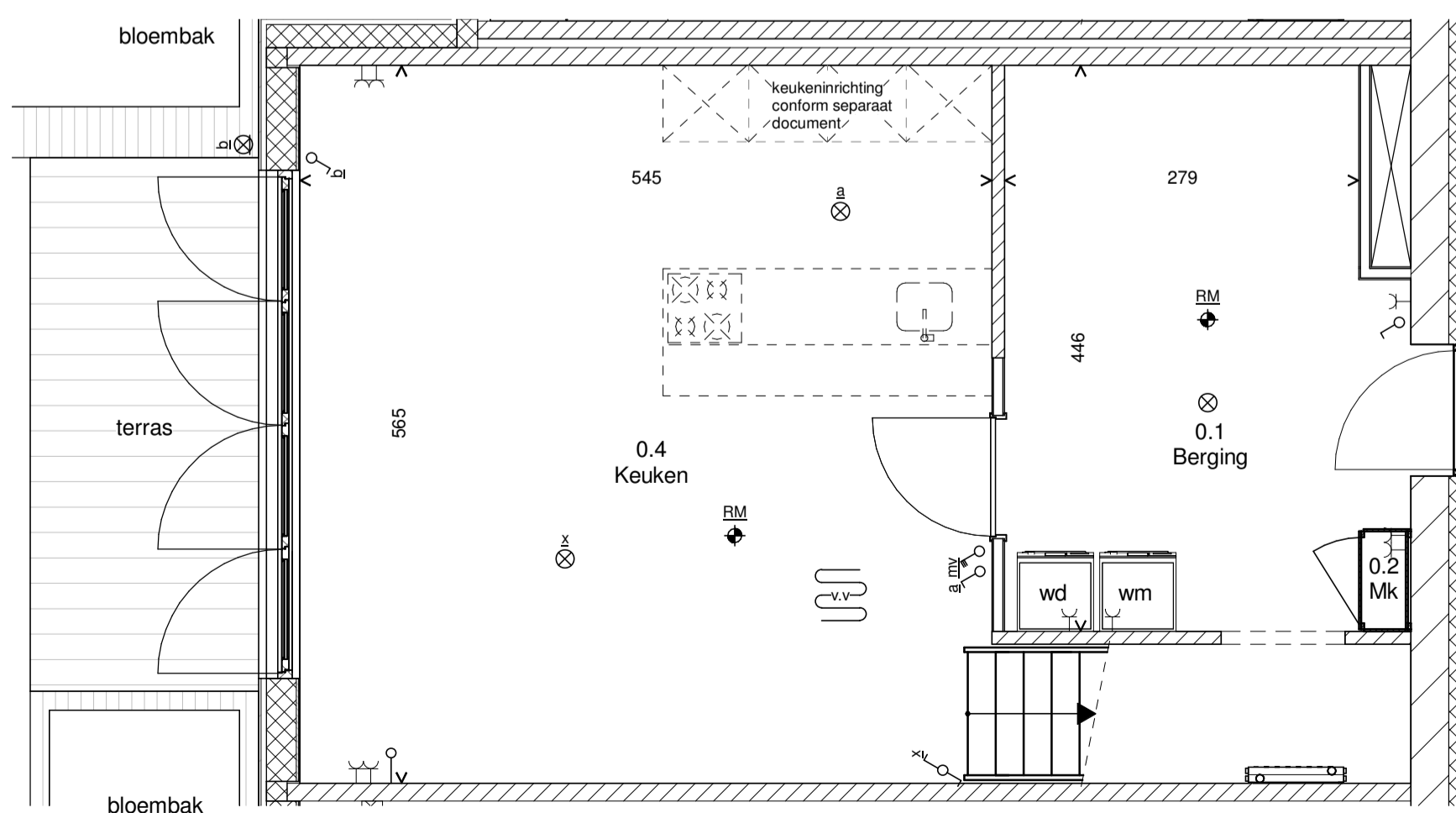
Begane grond
