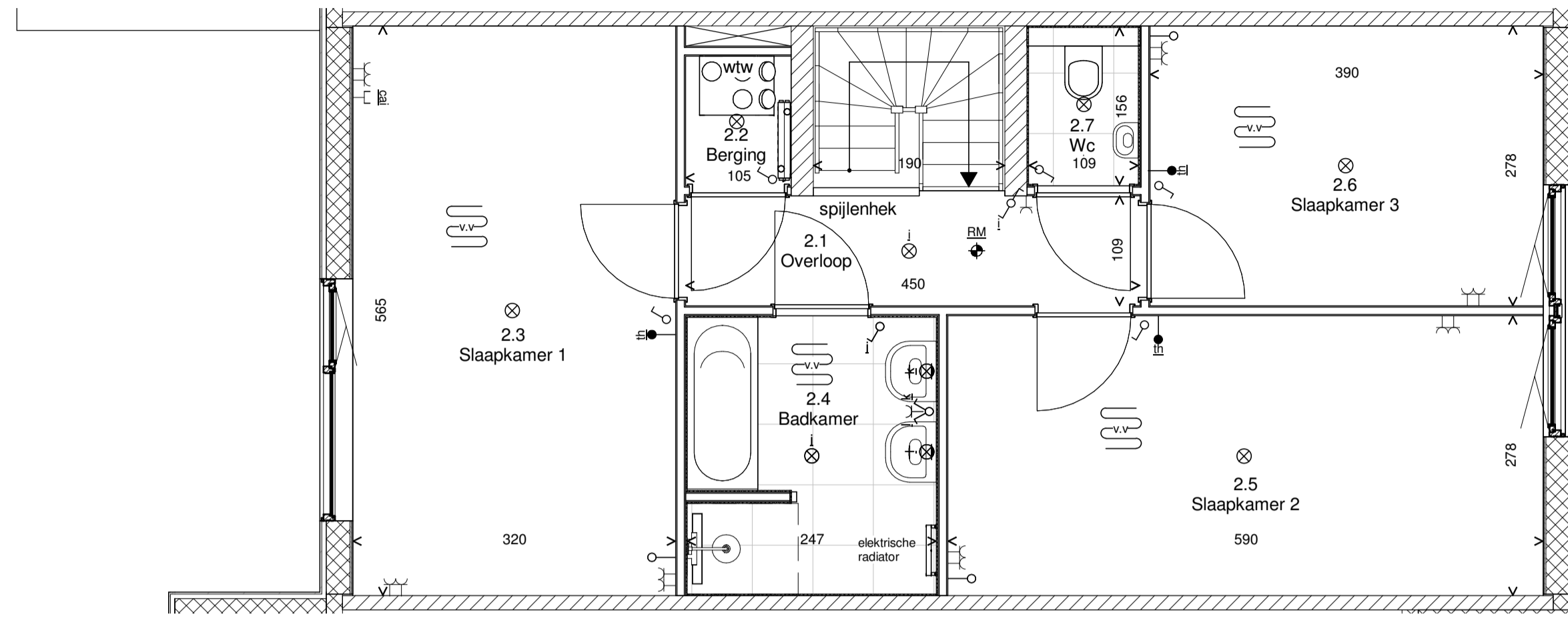
Tweede verdieping
