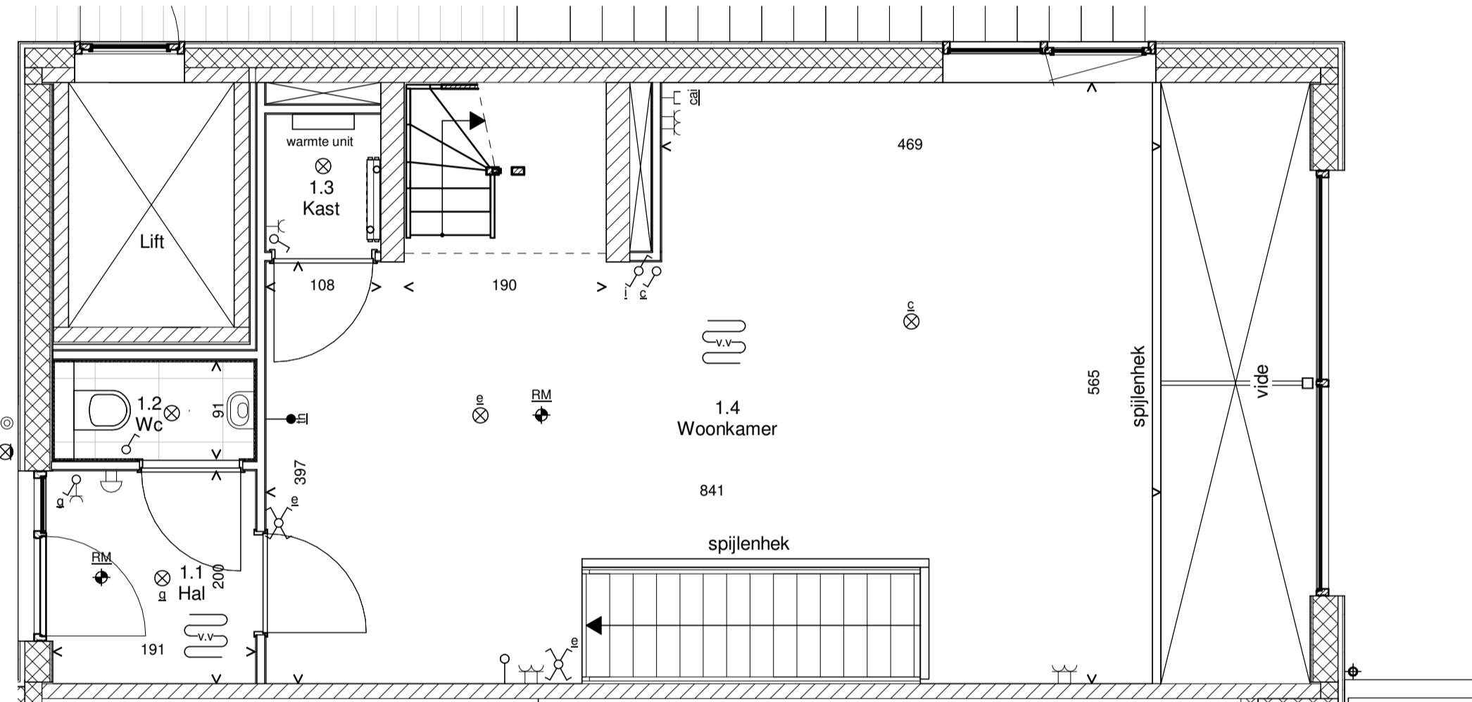
Eerste verdieping
