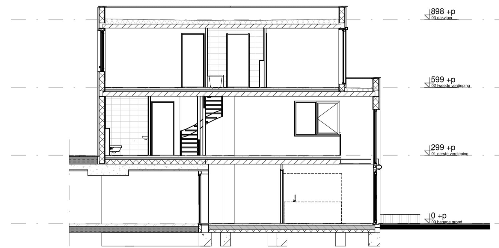
Doorsnede
