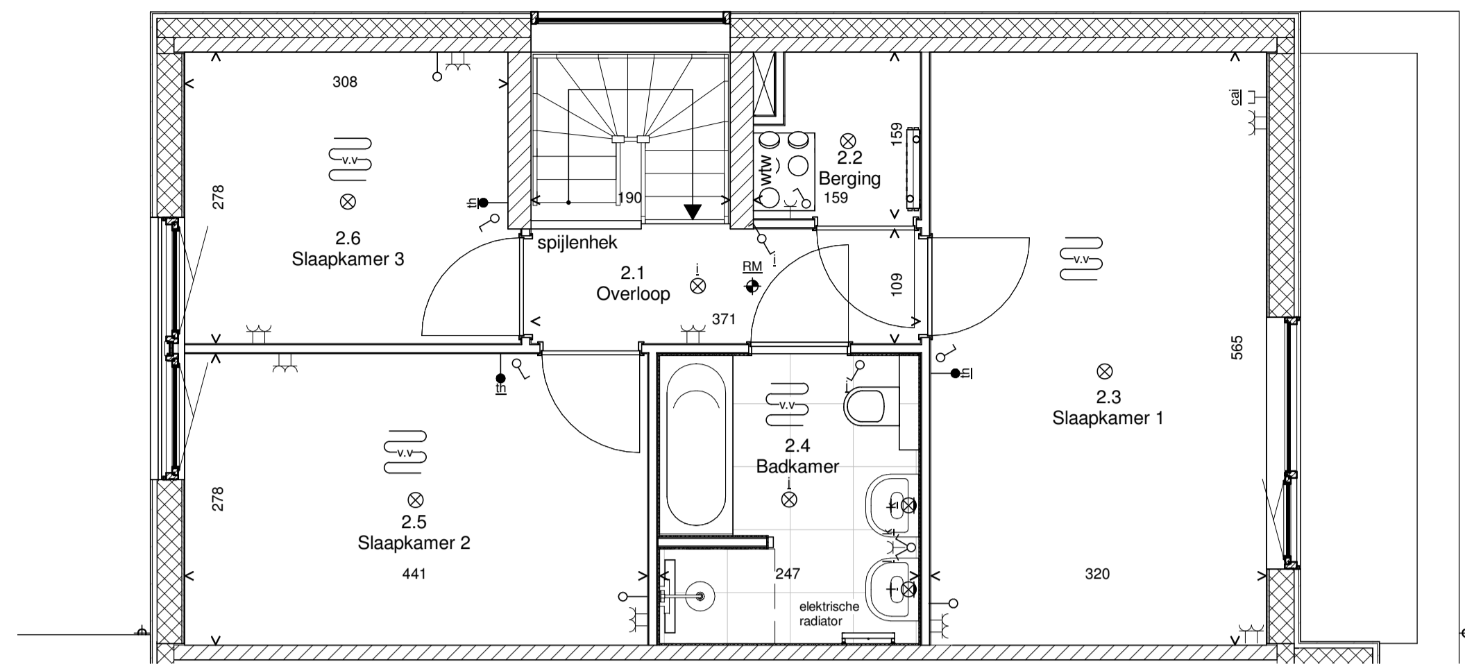
Tweede verdieping
