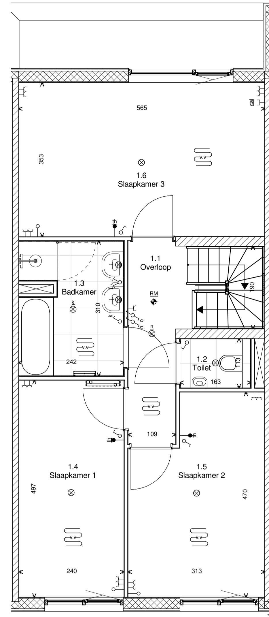
Eerste verdieping
