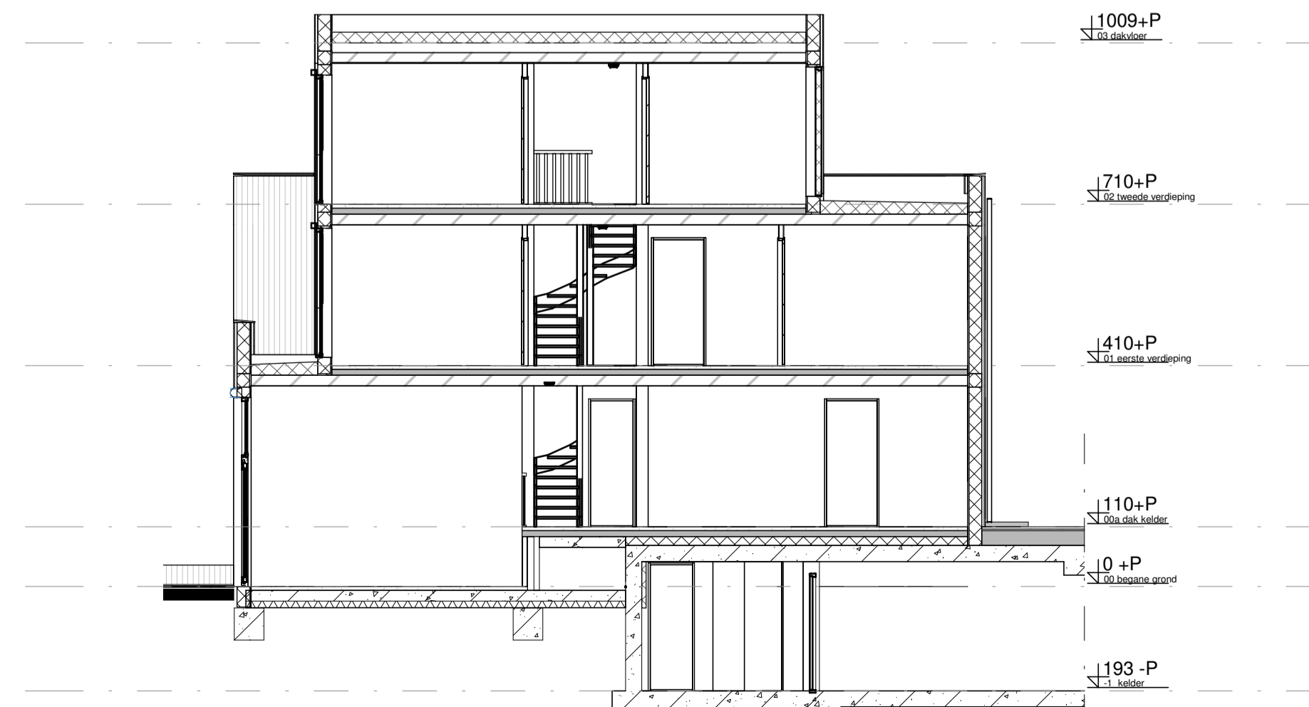
Doorsnede
