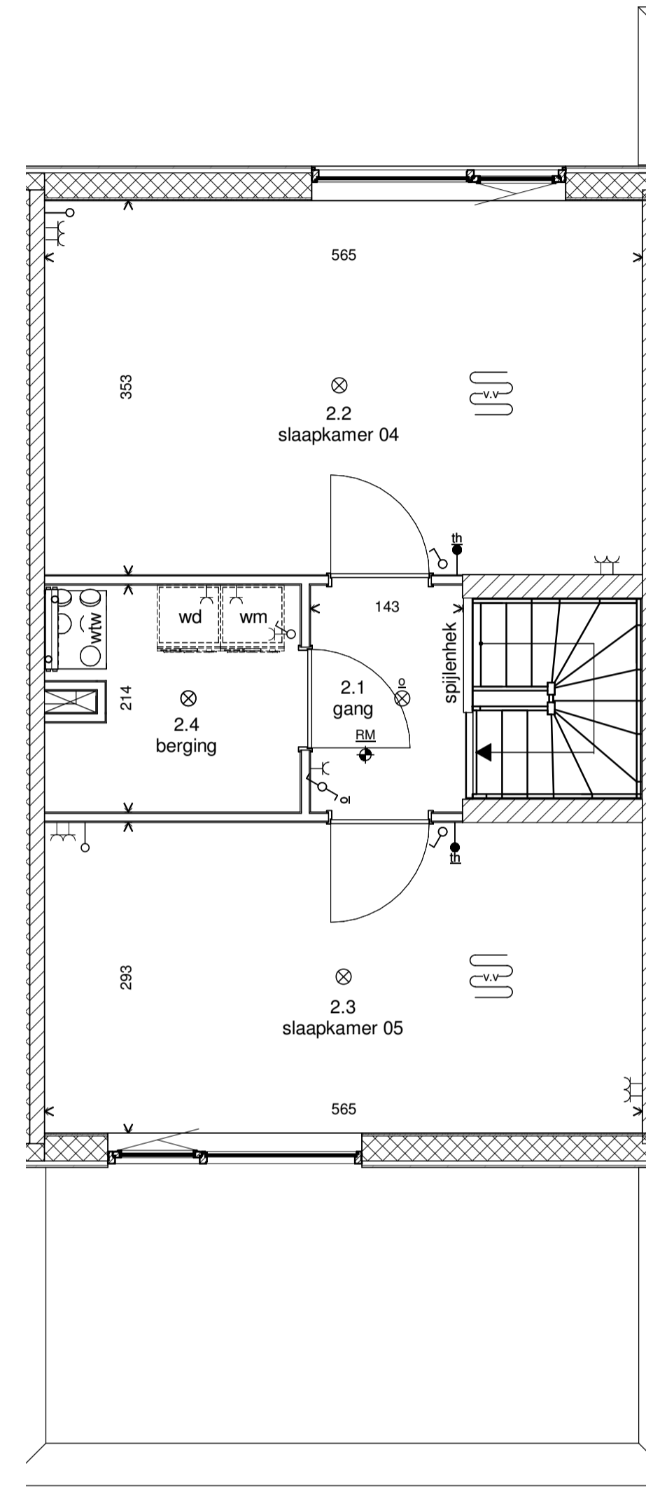
Tweede verdieping
