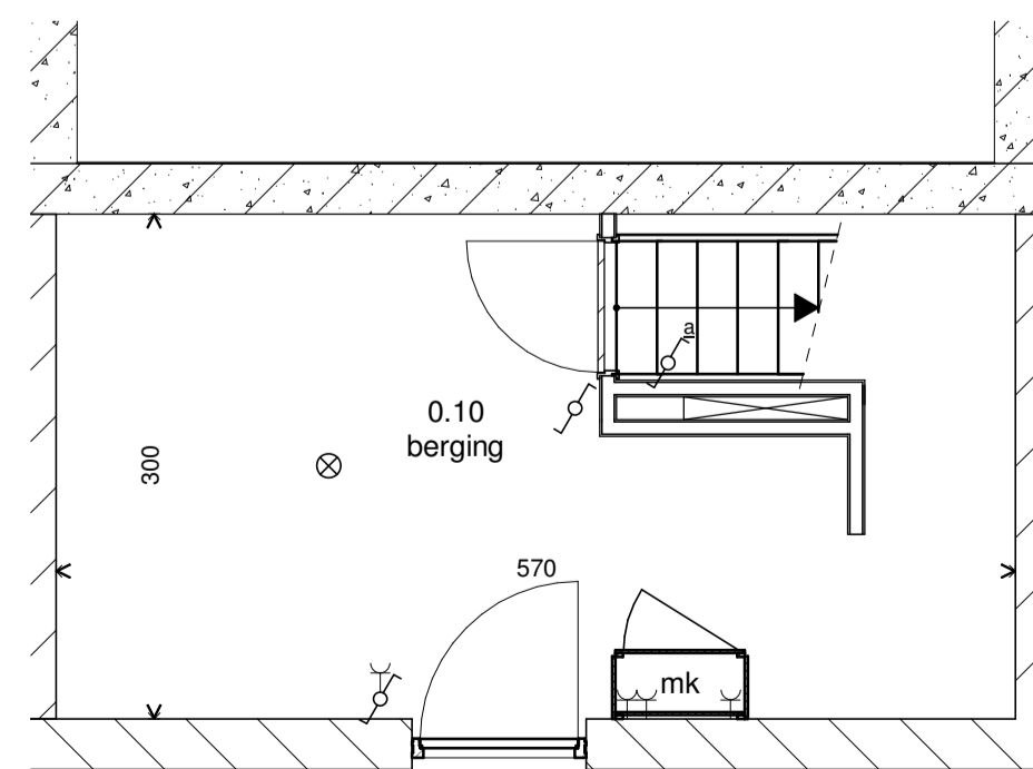
Kelder
