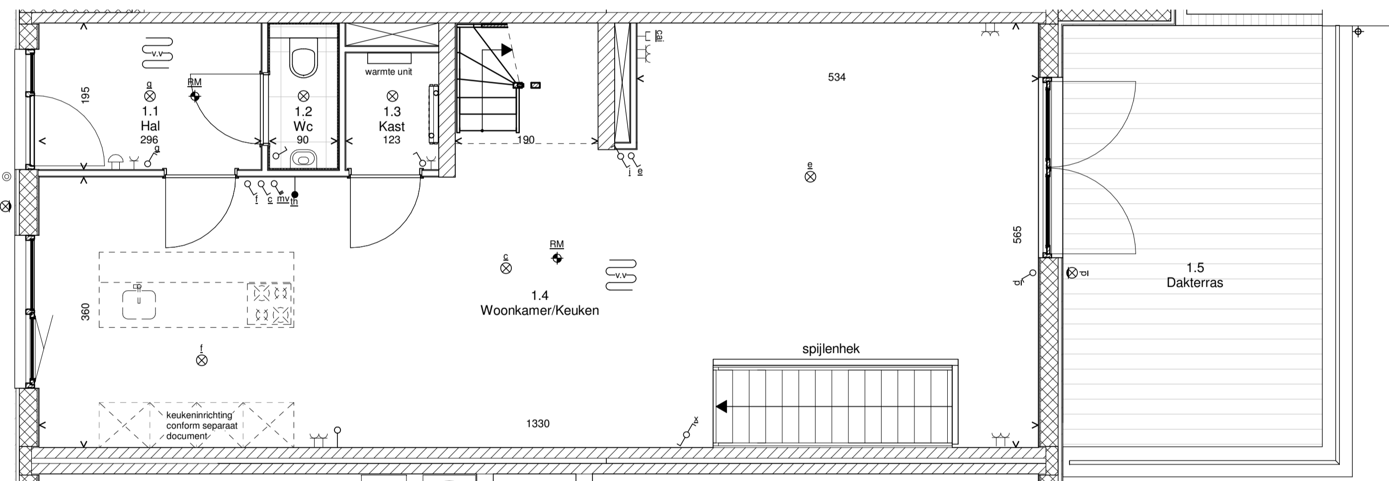
Eerste verdieping
