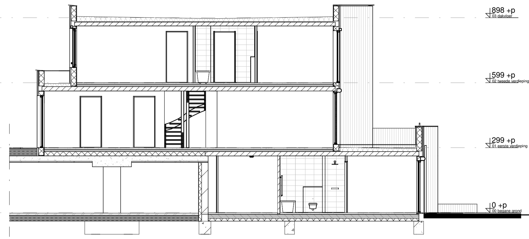
Doorsnede
