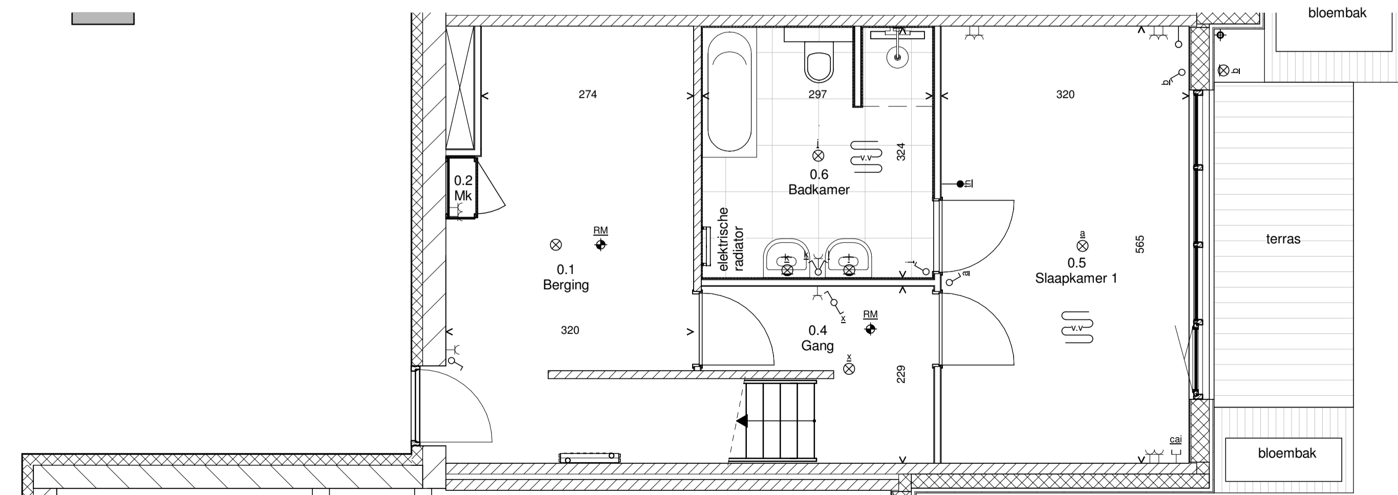
Begane grond
