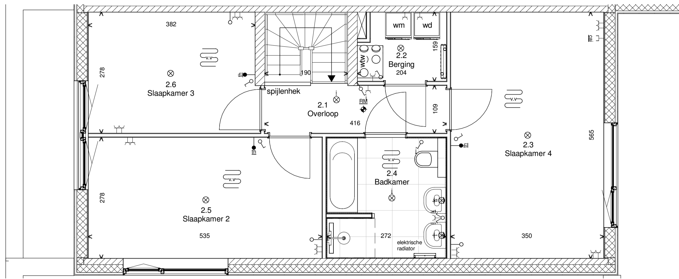
Tweede verdieping
