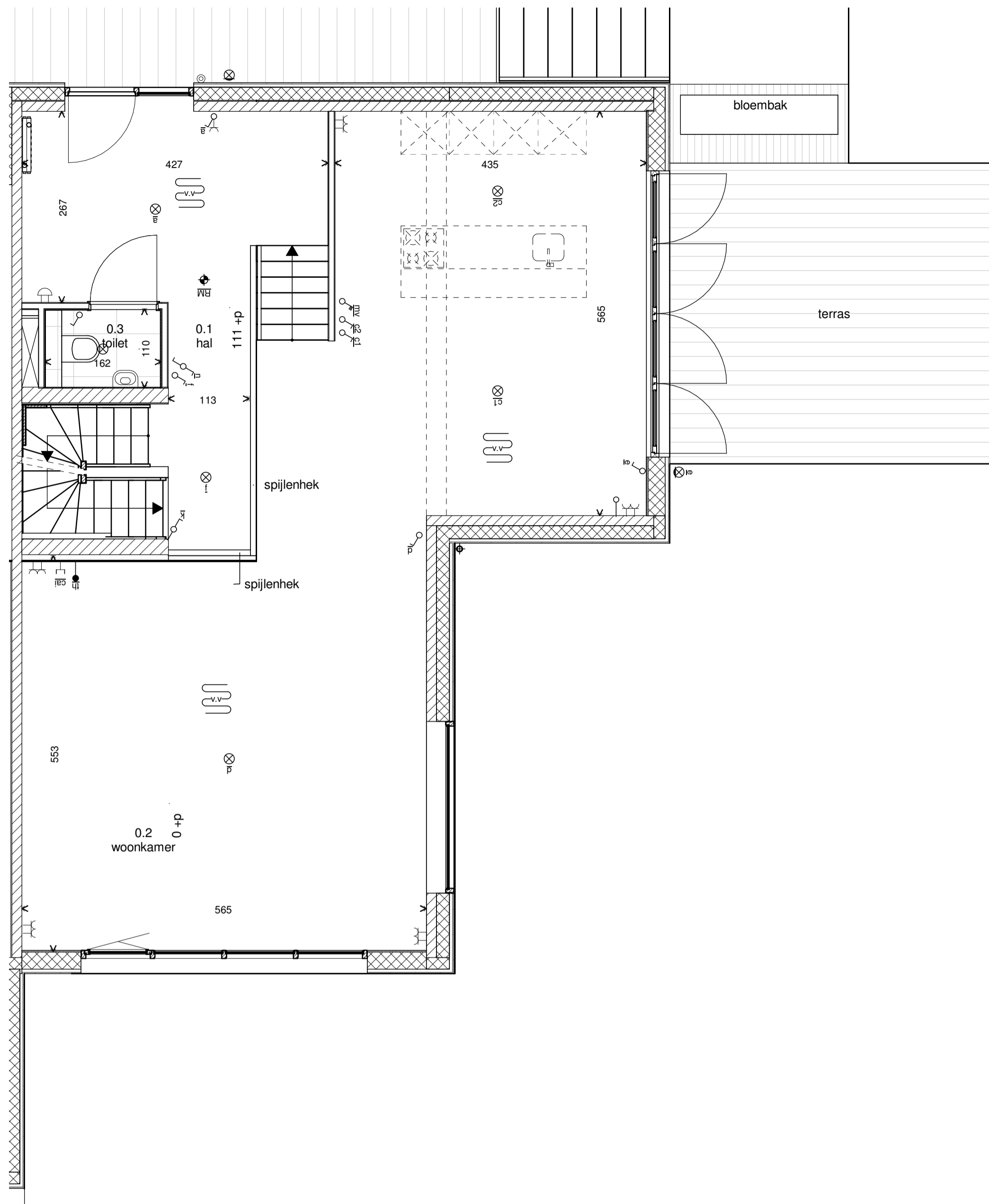
Begane grond
