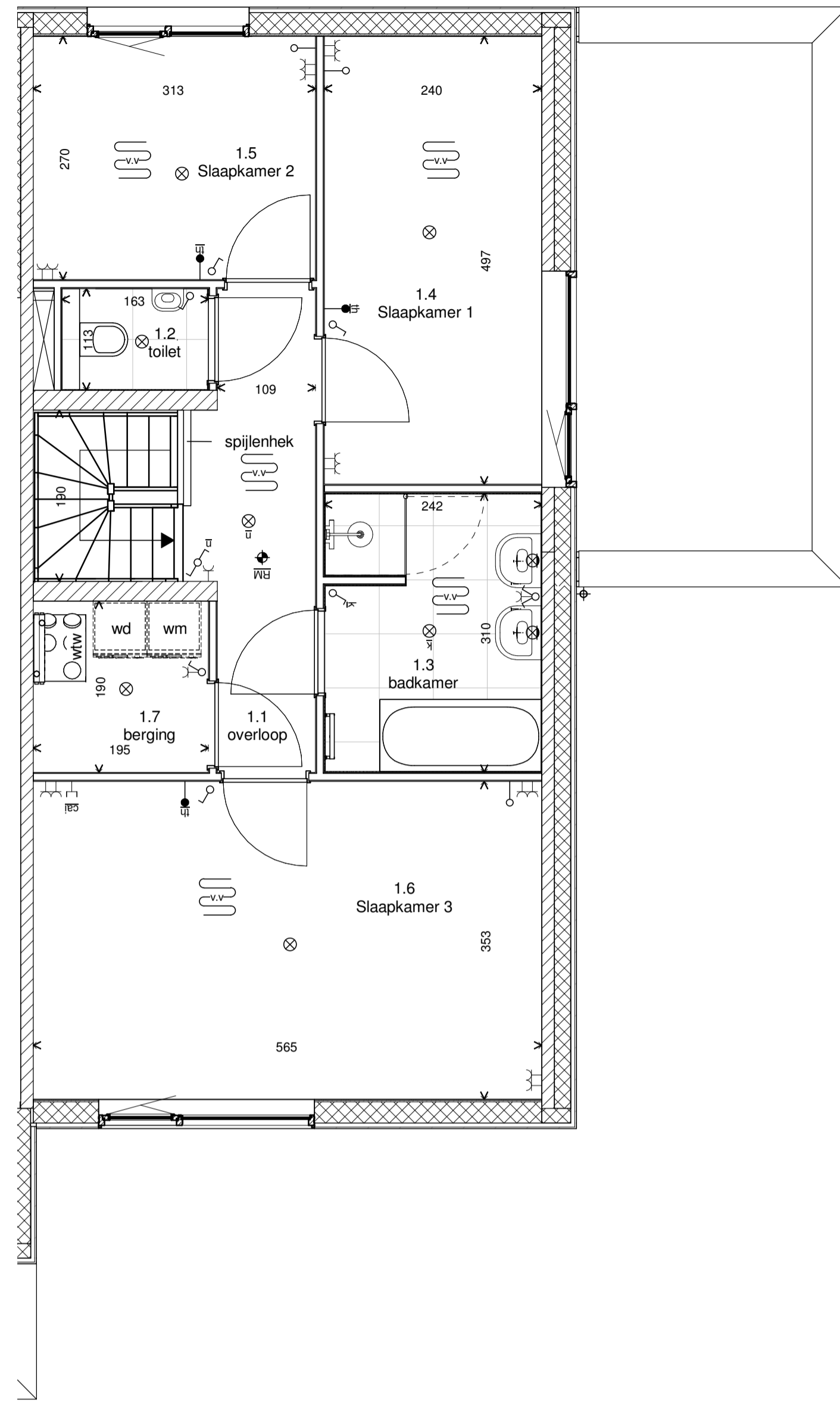
Eerste verdieping
