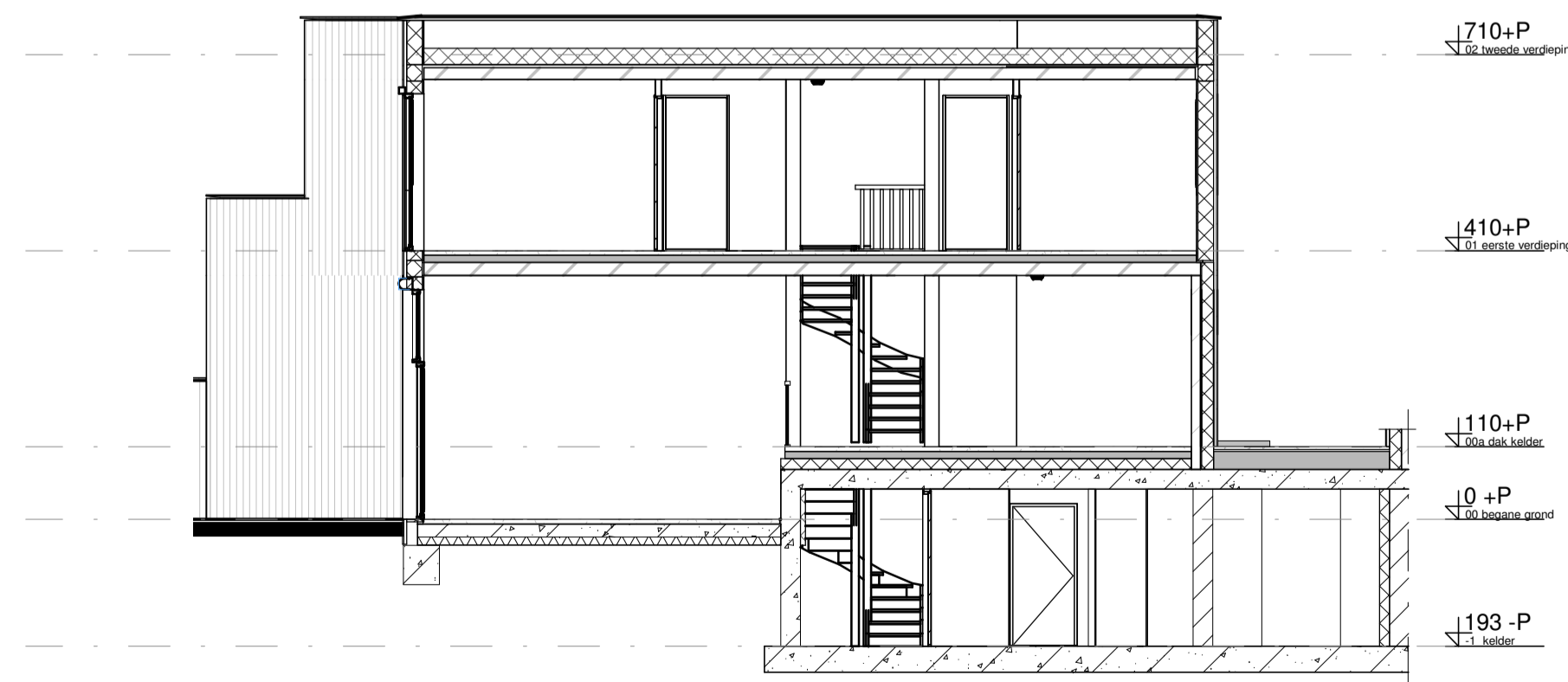
Doorsnede
